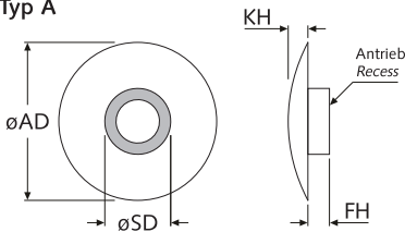
Schutzkappen für Inbus-Schrauben Screw caps for hexagon socket screw drive
