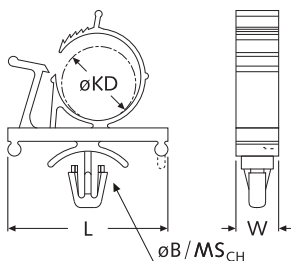
Rundkabelhalter, steckbar Plug-in round cable holders
