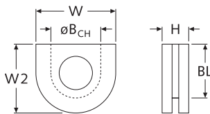
Membrantüllen, mit Rand, geschlossen/ geschlitzt/offen Membrane grommets with flat edge, closed/cut/open
