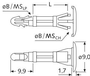
Flachkopf-Distanzhalter, universal, für drei verschiedene Bohrungen
